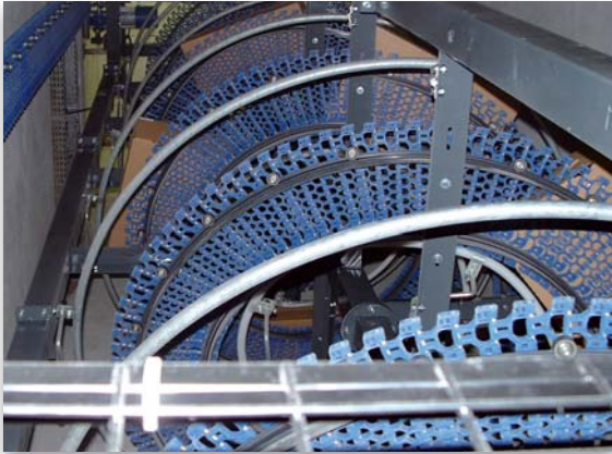
Ligne d'emballage avec descente de cartons à - 7 m (Spirale avec convoyeur modulaire)
